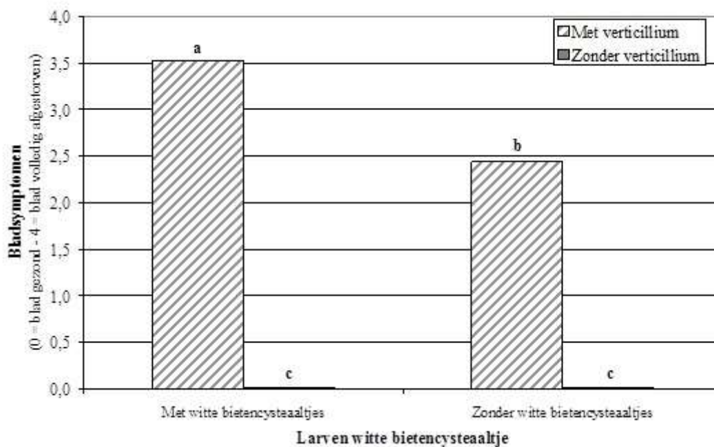
Figuur 10.5.13 Resultaat van een klimaatkamertoets naar het effect van het wit bietencysteaaftje op de mate van aantasting door verticillium. Waardering van bladsymptomen op een schaal van 0 (bladeren gezond) tot 4 (alle bladeren volledig afgestorven). Gemiddelde voor vier verticilliumisolaten en twee rassen. De verschillende letters boven de kolommen geven statistisch betrouwbare verschillen weer ( P < 0,001 ; kleinste significante verschil (5%) = 0,49).
