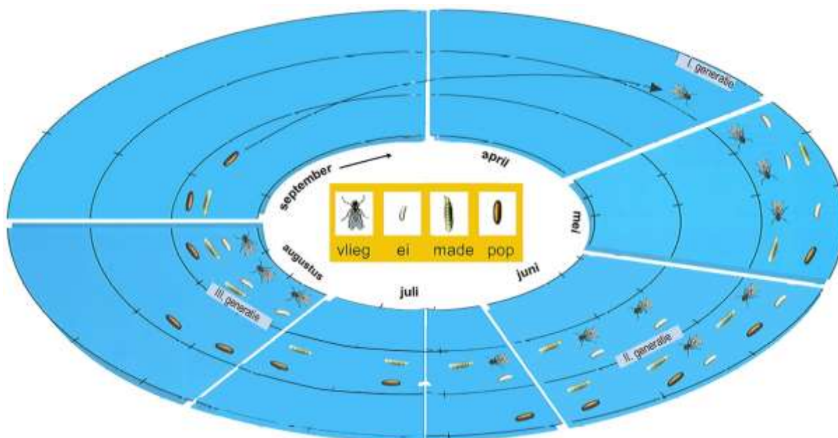
Figuur 10.3.8 Schematische weergave van de levenscyclus van de bietenvlieg (naar Brendler et al. , 2008 2 ).
