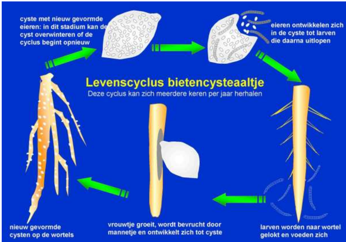
Figuur 10.2.7 Levenscyclus van het wit bietencystealtje.
